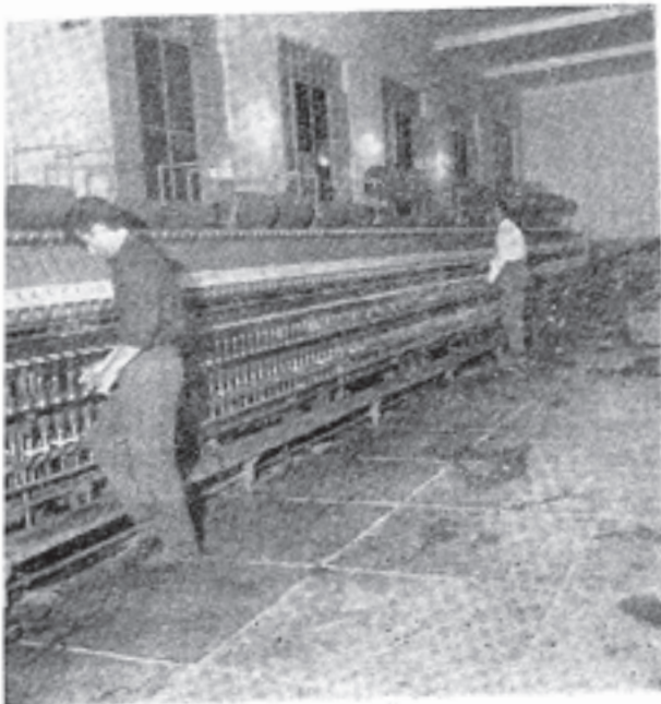
قسمتی از ماشین آلات ریسندگی کارخانه پشمیافی شرق
